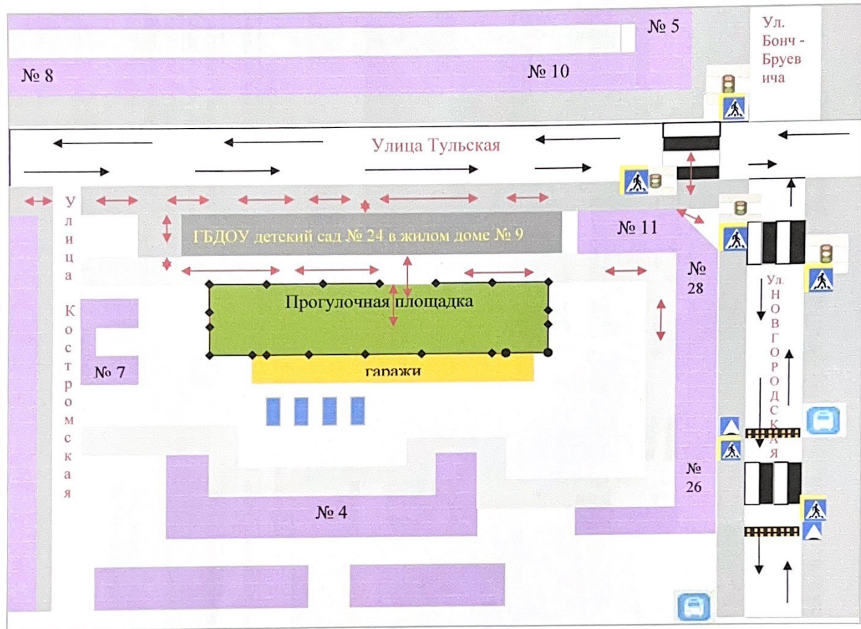
2. Схема организации дорожного движения в непосредственной близости от образовательного учреждения на ул. Тульской, д.9 с размещением соответствующих технических средств, маршруты движения детей и расположение парковочных мест
